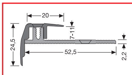
Typ PF 420 L (7 - 11 mm)
