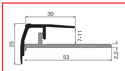
Typ PF 521 L (7 - 11 mm)
