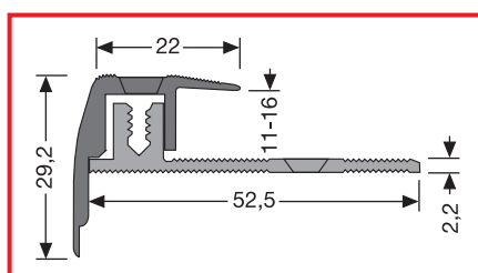
Typ PF 420 (11 - 16 mm)
