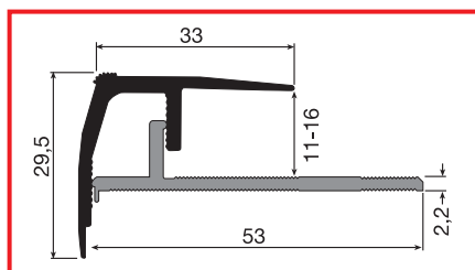
Typ PF 521 (11 - 16 mm)
