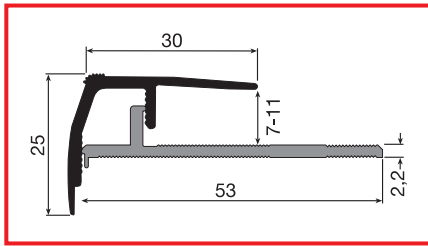
Typ PF 521 LH (7 - 11 mm)
