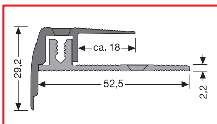
Typ PF 421 (11 - 16 mm)
