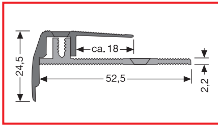
Typ PF 421 L (7 - 11 mm)
