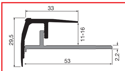
Typ PF 521 H (11 - 16 mm)
